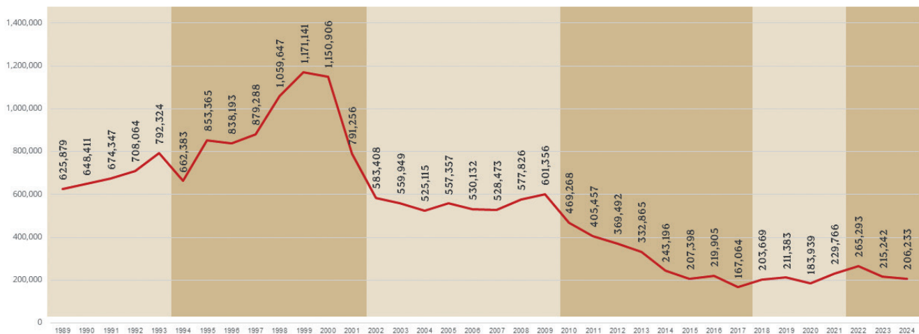
Gráfica 1. Mexicanas y mexicanos repatriados desde Estados Unidos (1989 a 2024)
